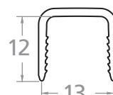
SE-1312 SPEED 13x12x12mm
